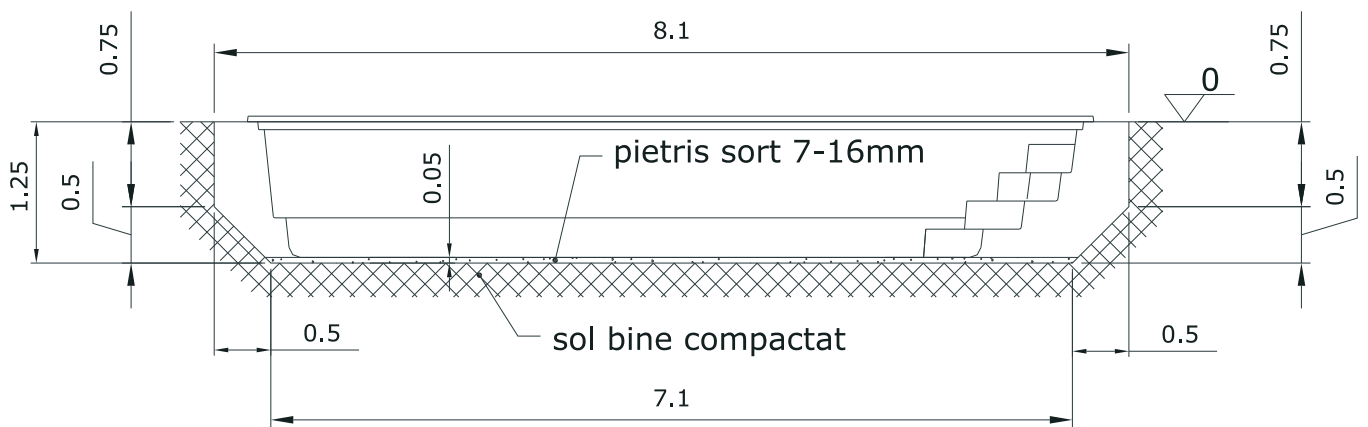
Secțiunea A-A
