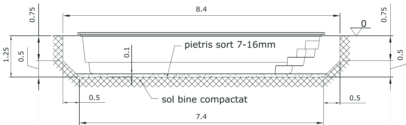
Sectiunea A-A
