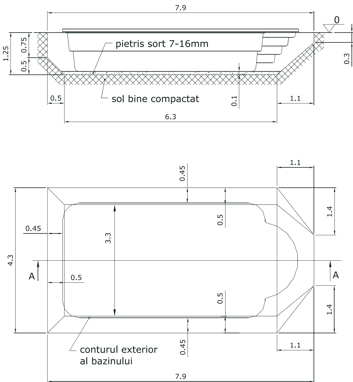
Sectiunea A-A
