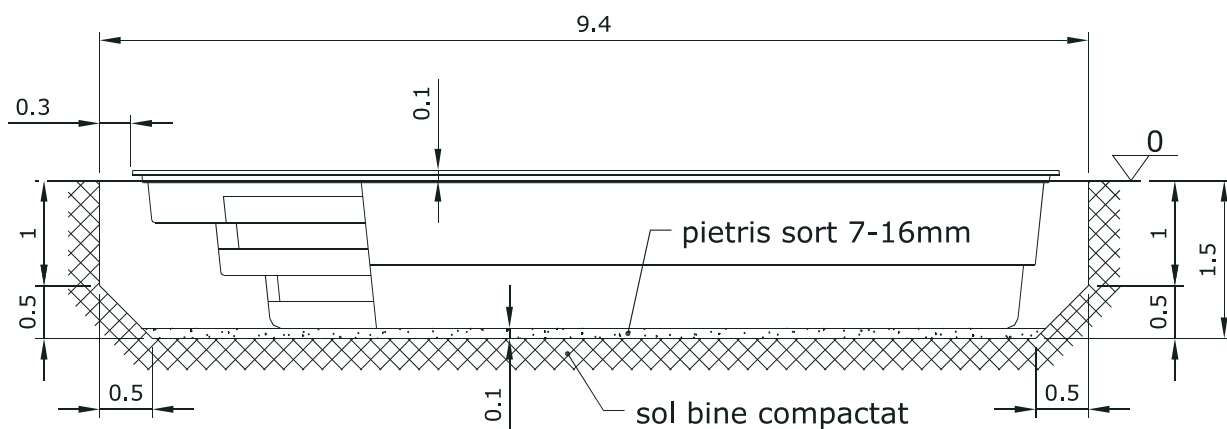
Sectiunea A-A
