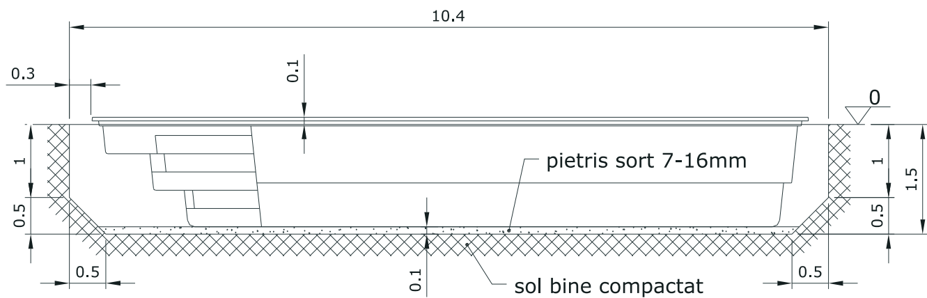
Sectiunea A-A
