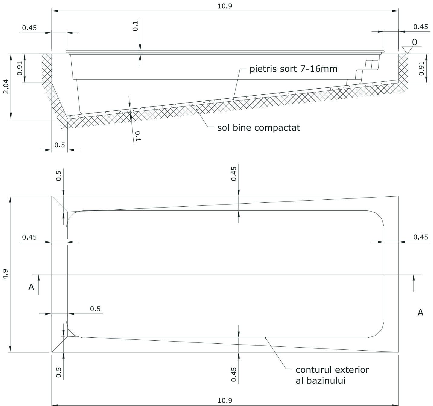
Sectiunea A-A
